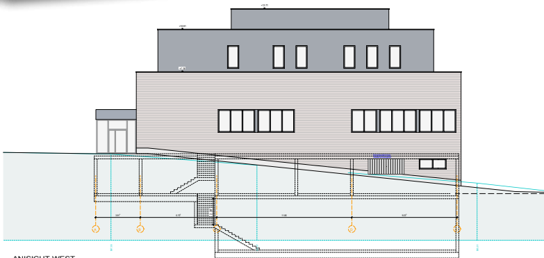
ANISICHT WEST
