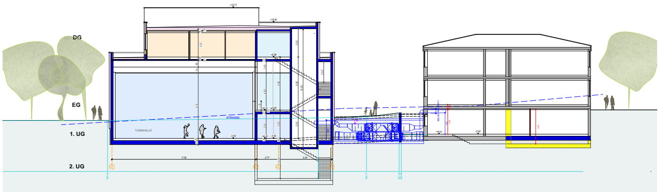
SCHNITT 2
